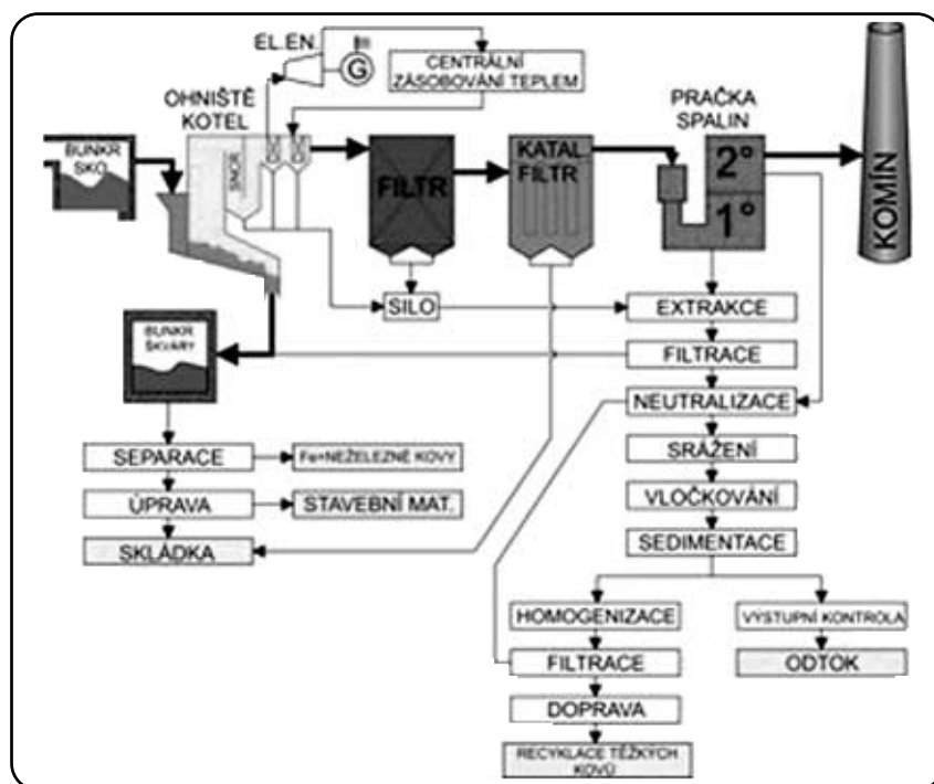
Obr. 1: Příklad technologického řetězce spalovny s odvodem vyčištěných pracích vod / Zdroj: www.odpadjeenergie.cz, E.I.C., spol. s.r.o.
